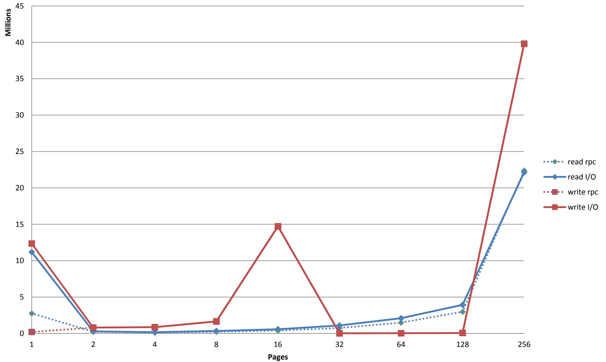
Pages per RPC and disk I/O
